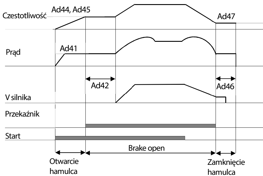
Algorytm V/f
